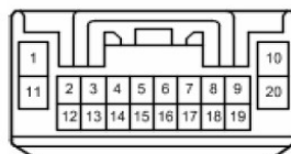
GE1コネクタ
